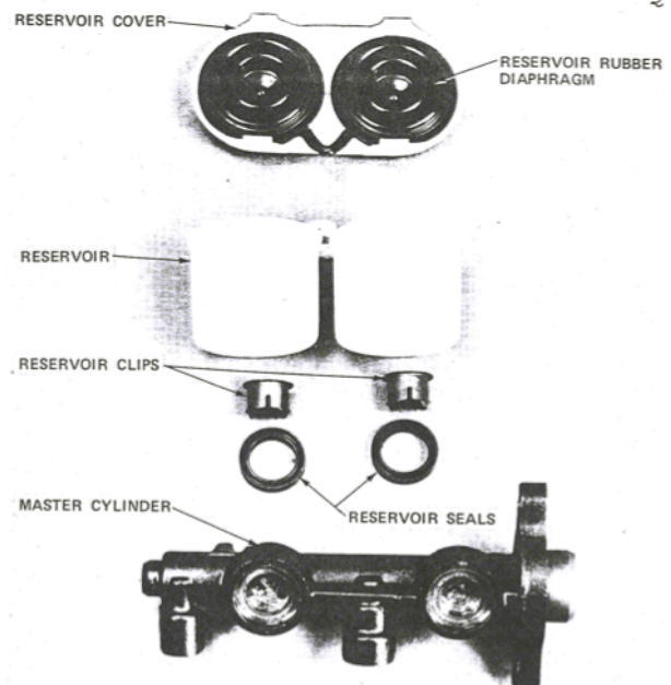
Einzelteile des Behälters und Innenansicht Deckel
